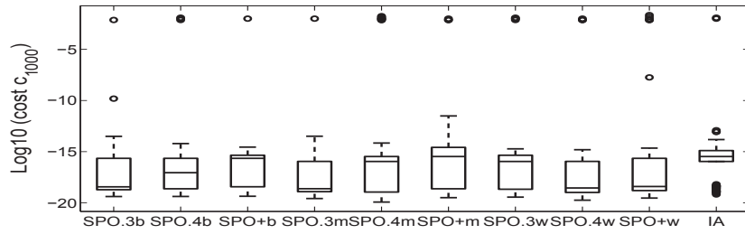
(d) CMAES-Griewangk
