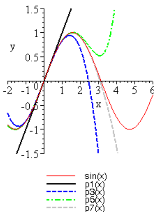
Abbildung 5-3: Approximation der Sinus-Funktion durch seine Taylorpolynome im Punkt x=0 .
