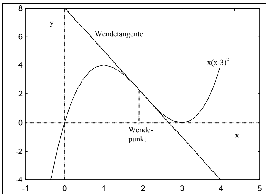
Abbildung 5-6: Wendepunkt x = 2 und Wendetangente an die Funktion x(x-3)^2
