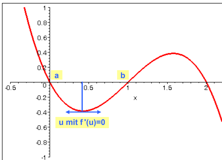
Abbildung 5-2: Graph der Funktion -x(x-1)(x-2) zur Erläuterung des Mittelwertsatzes
