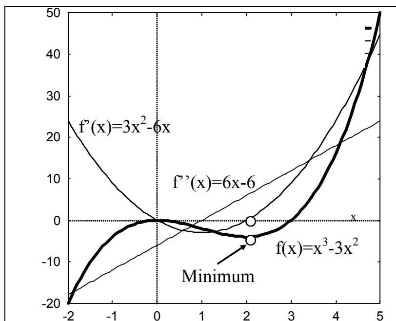
Abbildung 5-4: f(x) = x^3 - 3x^2 mit 1. und 2. Ableitung
