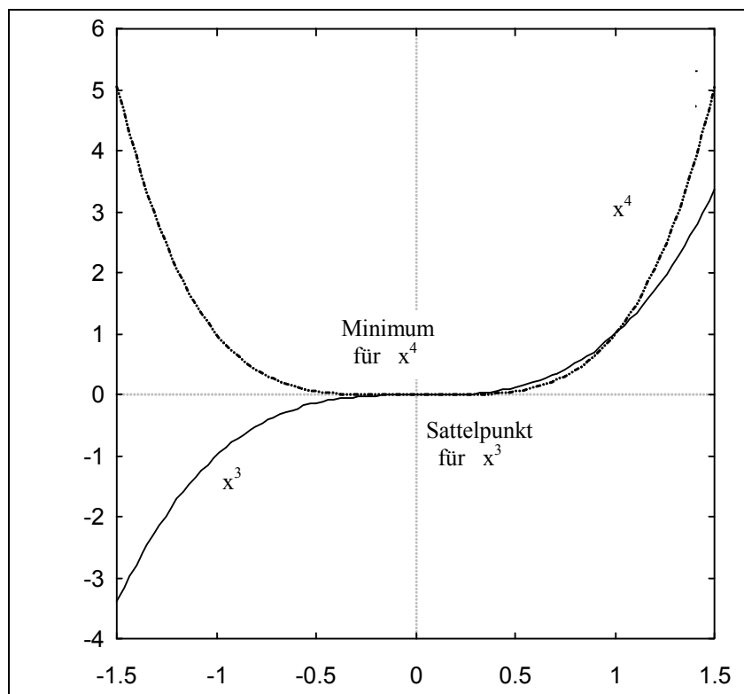
Abbildung 5-5: Veranschaulichung von x^3 mit Sattelpunkt bei x = 0 und x^4 mit Minimum bei x = 0
