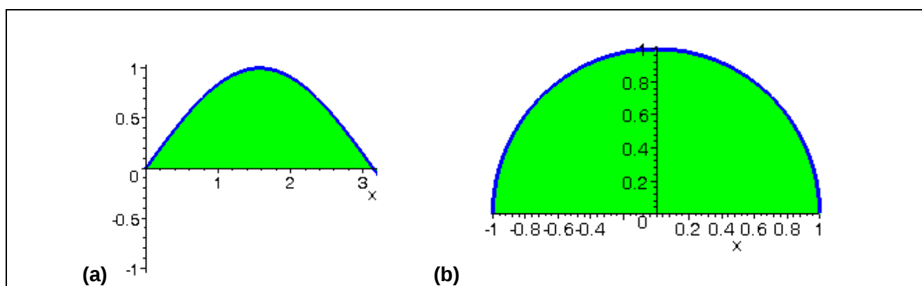
Abbildung 6-2: Weitere Integrale
