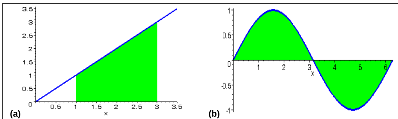
Abbildung 6-1: Geometrisch berechenbare Integrale
